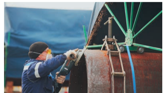
Вырезка технологических окон и обработка кромок трубы — не самые зрелищные, но одинаково важные моменты конкурса
