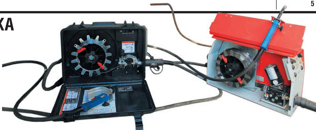
С новой технологией сварщику уже не нужно постоянно менять электроды: его «электрод» — катушка с самозащитной проволокой в подающем устройстве
